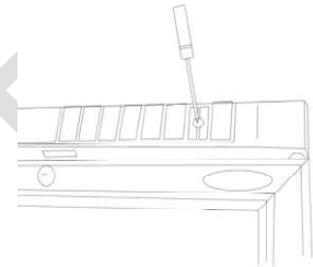
3. Toppanel/Canopy afmonteres.
