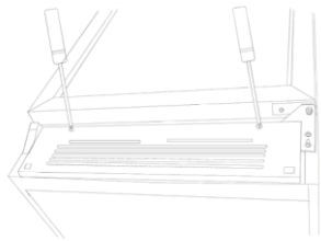
1. Bundpanel afmonteres.
